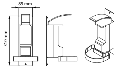
Sanitizer Dispenser Vol1 - 0,5 L
