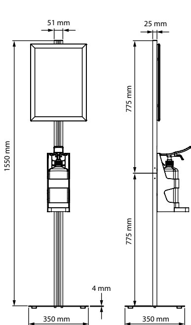
Sanitizer Dispenser Vol1 - 0,5 L
