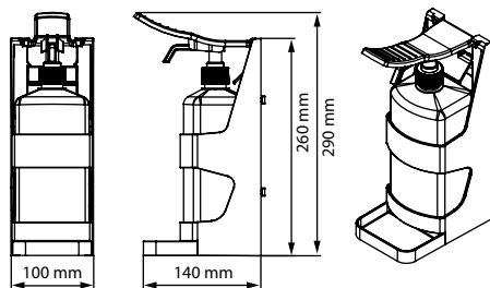
Dispenser Vol2
