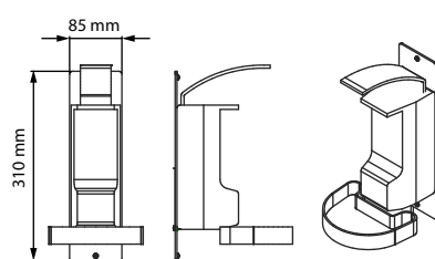
Sanitizer Dispenser Vol1 - 0,5 L
